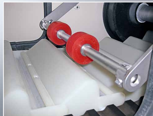
Pendelklopper zur Unterstützung des Produktauswurfs
