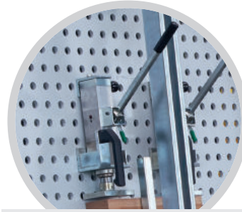
Handhydraulikzylinder fest, mit 2 Rastbolzen Fixed manual hydraulic cylinder, with 2 matrix bolts
