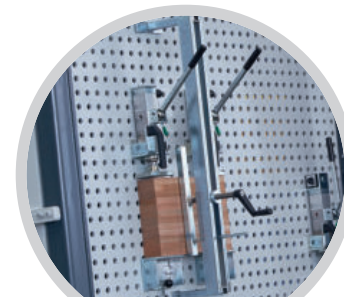
Niederhalter kurz, 800 mm, mit Spindelklemmung Side pressure clamp, 800 mm, spindle driven
