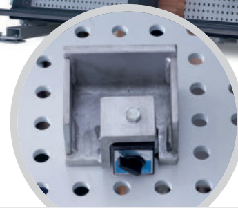
Einzelaufgabe 360° schwenkbar, mit Magnetfeststeller Single support, rotatable by 360°, magnetic lock
