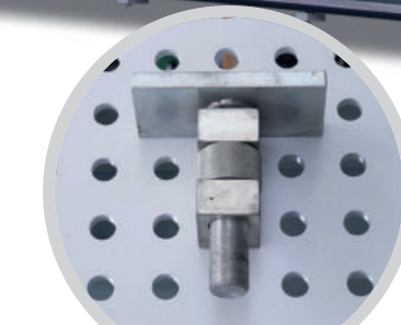
Einzelaufgabe fest, maßestellbar Fixed single support, adjustable
