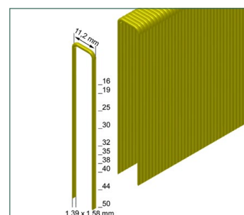
Abmessungen Type Z
