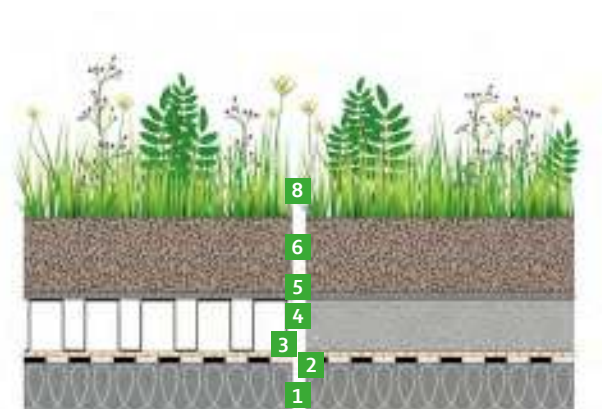
Abb. 39: Schematische Darstellung einer mehrschichtigen Dachbegrünung. Quelle: BuGG
