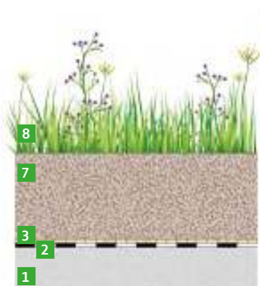
Abb. 38: Schematische Darstellung einer einschichtigen Dachbegrünung. Quelle: BuGG
