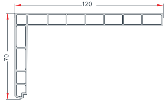
7 X 12 CASING PROFILE 7 x 12 PERVAZ PROFİLİ EN 51
