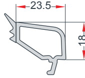
18-mm DOUBLE GLAZING BEAD 18 mm ÇİFT CAM ÇİTASI EN 41
