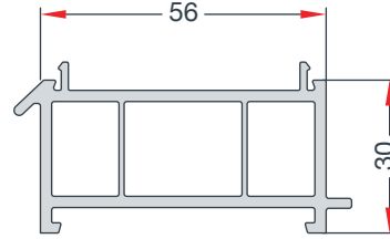
30 x 56 EXTENDER PROFILE 30 x 56 YÜKSELTME PROFİLİ EN 114 HIGHLINE
