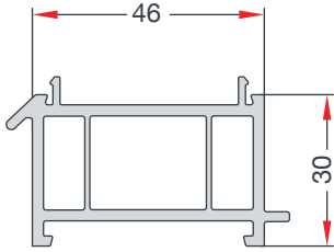
30 x 46 EXTENDER PROFILE 30 x 46 YÜKSELTME PROFİLİ EN 113 KLASLINE
