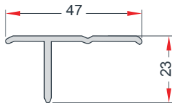
ASYMETRIC "T" PROFILE ASİMETRİK "T" PROFİLİ EN 64
