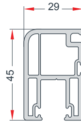
FLY SCREEN SASH PROFILE SİNEKLİK KANAT PROFİLİ EN 34
