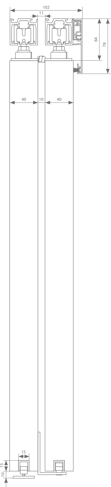
Parallele Deckenmontage 1
