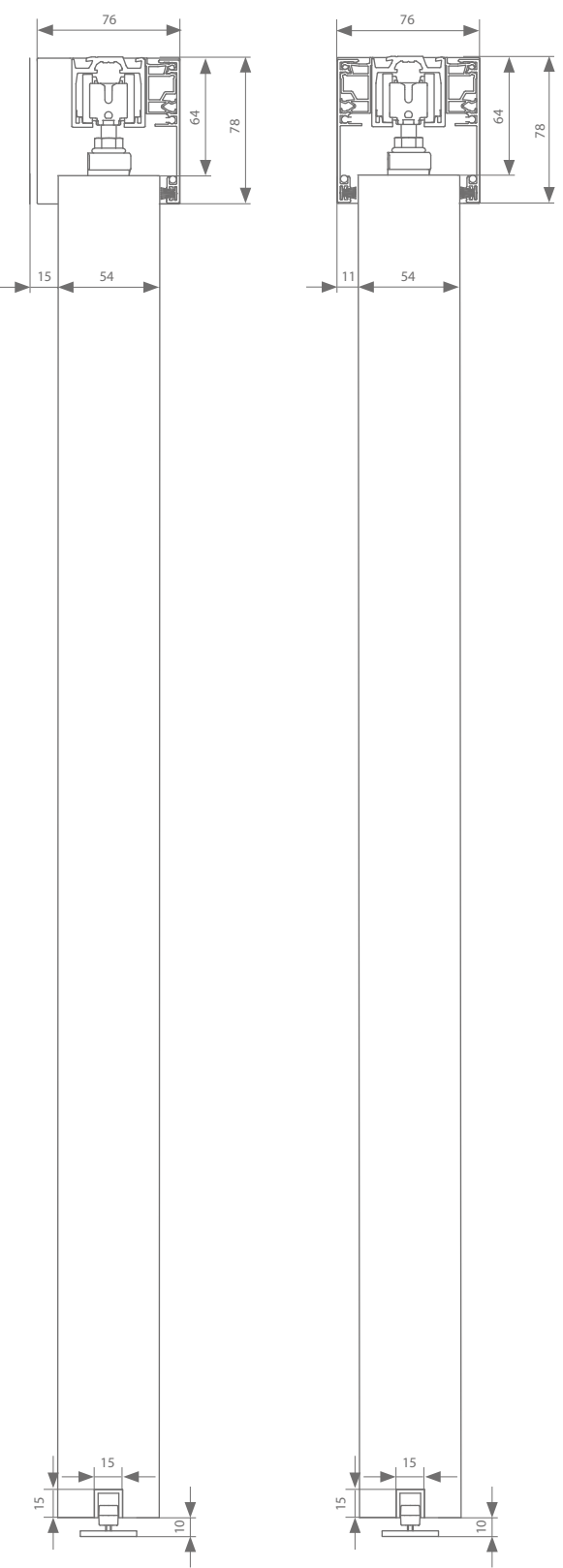
Deckenmontage 54 mm
