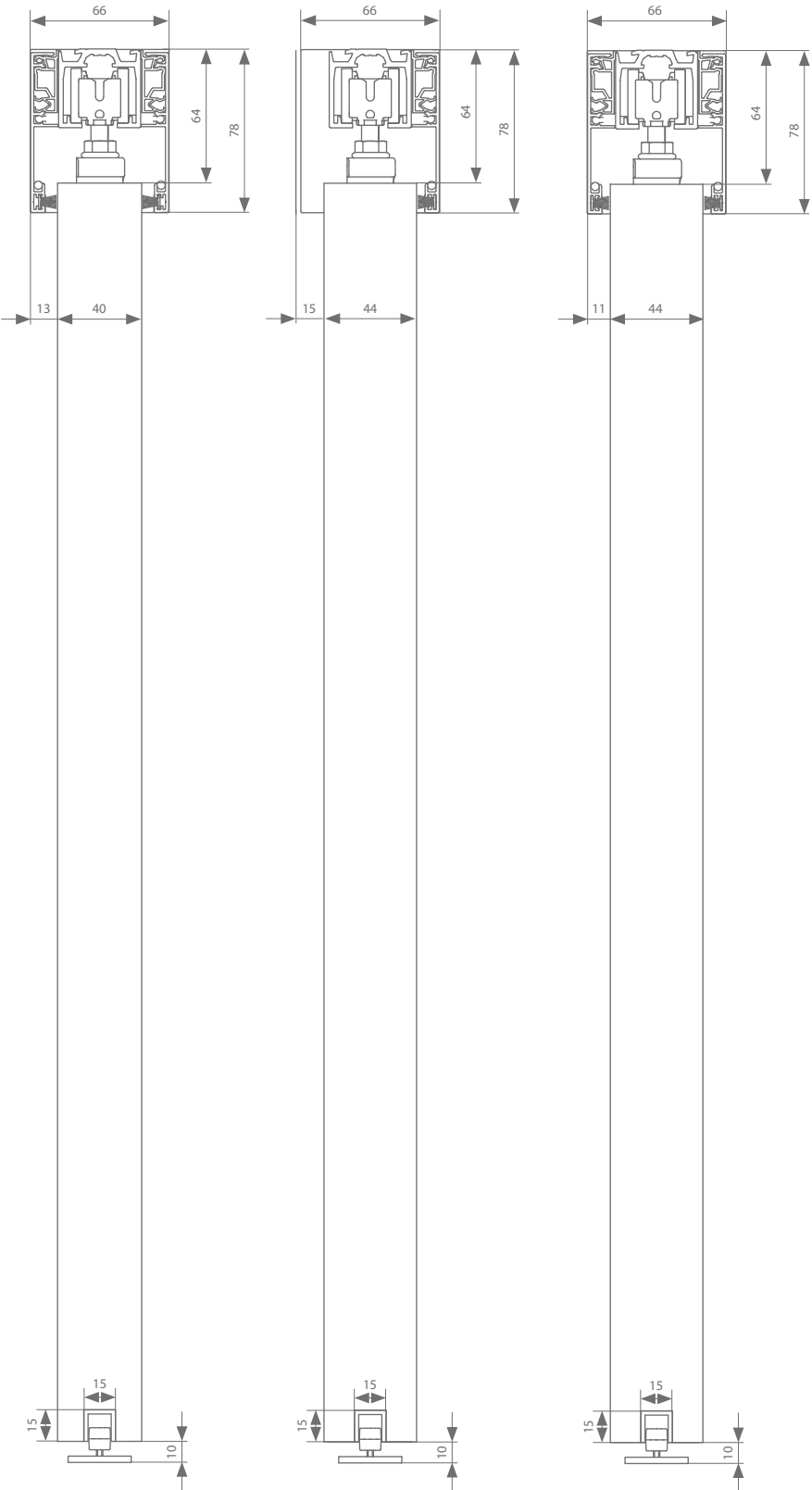
Deckenmontage 44 mm
