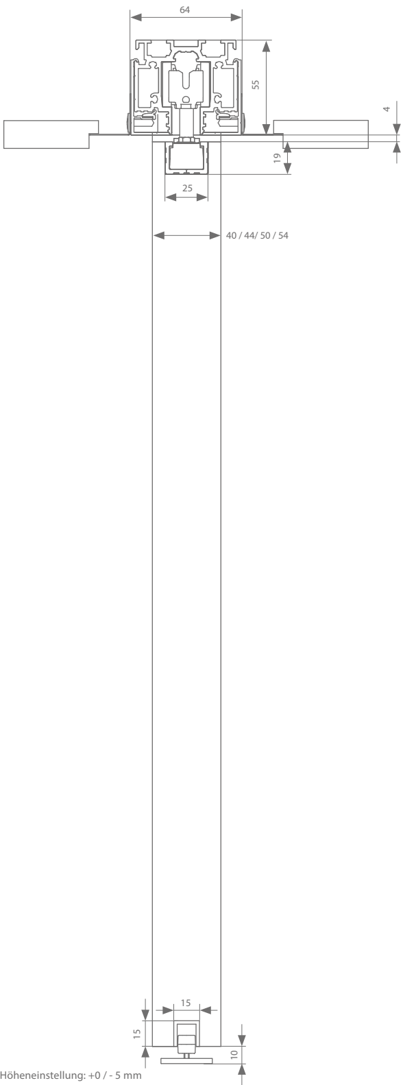
Für Systemdecke (1+2)
