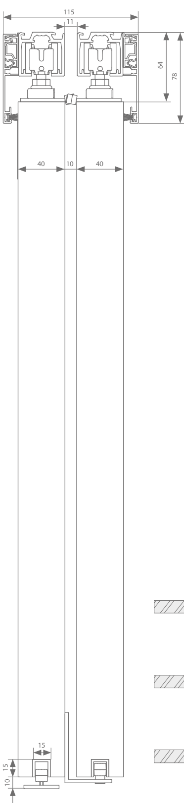
Parallele Deckenmontage 2
