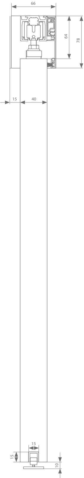
Deckenmontage 40 mm
