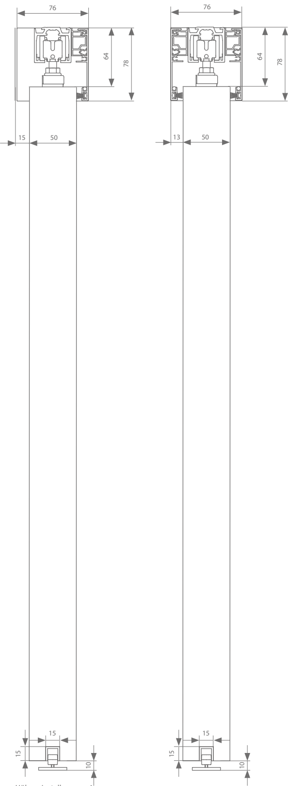
Deckenmontage 50 mm
