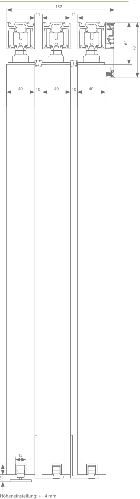
Parallel Deckenmontage 1
