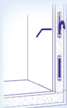
KRAFTSCHLÜSSIGE PANEELVERBINDUNG dank eingeschäumter Spannverschlüsse
