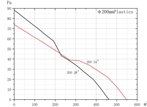
NEC4810/1800rpm
