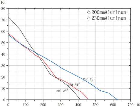
NEC4810/1500rpm
