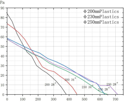
NEC4810/1500rpm
