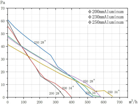
NEC4810/1300rpm
