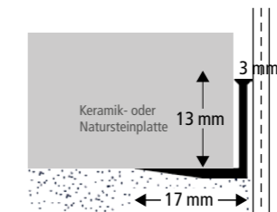
L-Profil für Fassandenanschluss
