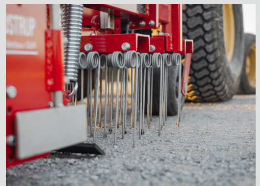
Federzinkenreihen & Kantenbrecher
