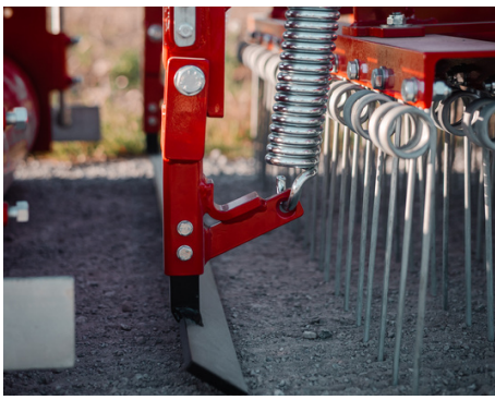
Unterschneidmesser
