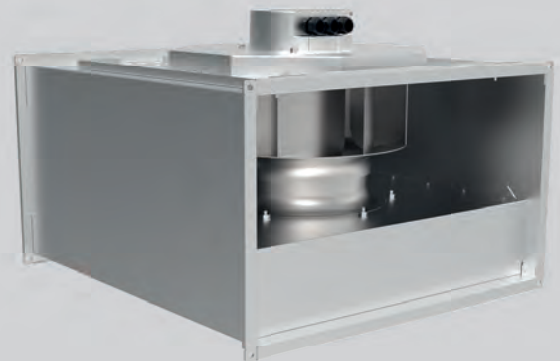
Kanalventilator (klappbar) für den Einbau in Kanalsysteme, z.B. Be- und Entlüftung von Gewerbe- und Industriegebäuden
