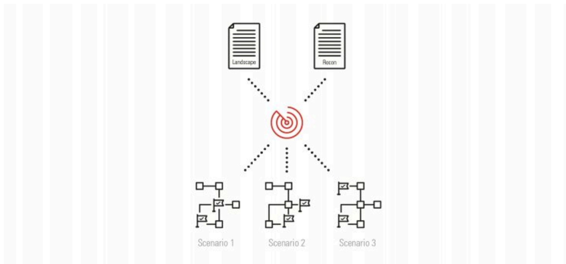
Figure 4.3: Module TI/SCENARIO
