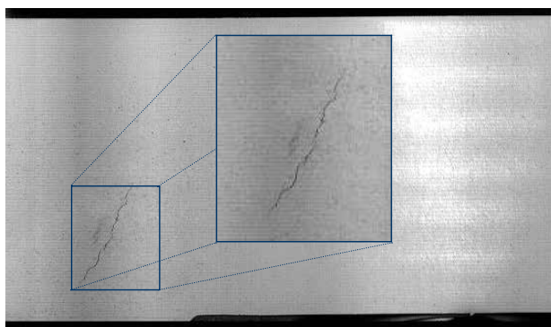
Riss auf einer Zylinderlauffläche
