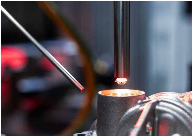
Optische Bohrungsinspektion
