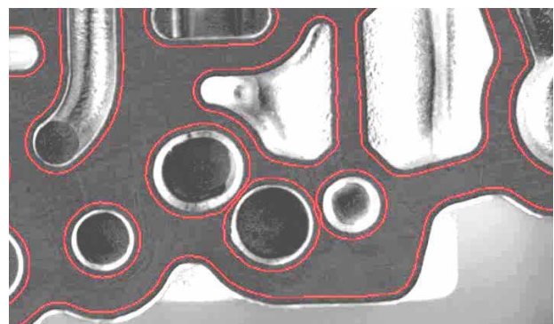
Kantengenaueres Prüfen dank adaptiver dynamischer Maskierung
