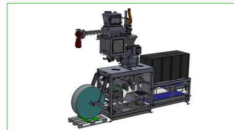
Automatische Schlauchfolienanlagen Automatic tubular FFS machines
