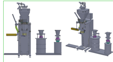
Trommel- und Fassfüller Drum- and pail fillers
