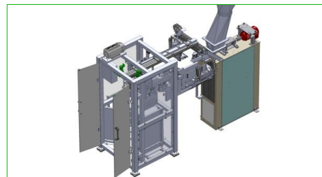
Automatische Ventilsackanlagen Automatic valve bag fillers
