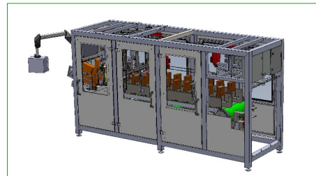
Absackautomaten für Klotzbodenbeutel Automatic fillers for block bottom bags
