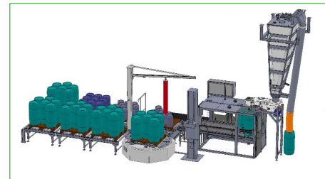
Automatische Fassfüllanlagen Automatic drum filling lines
