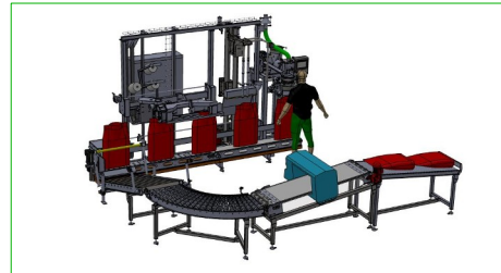
Halbautomatische Offensackanlagen Semi-automatic open mouth baggers
