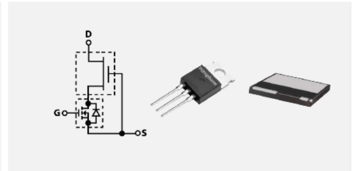
GaN HEMTs
