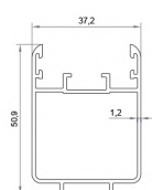
SUISS ESPAGNOLETTE LOCK PROFILE
