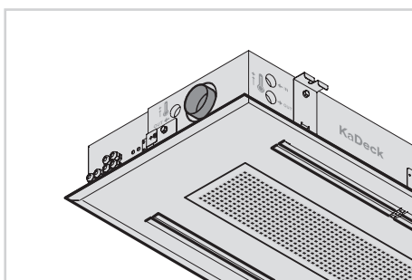
Primärluftstutzen Seitenansicht
