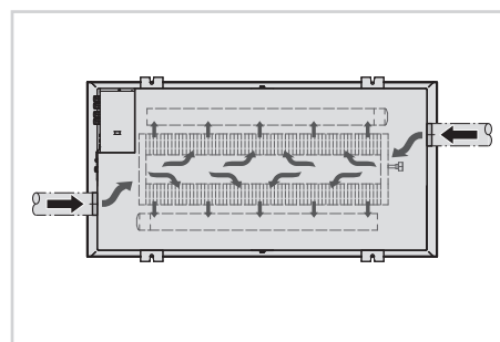
Primärluftstutzen beidseitig angeschlossen
