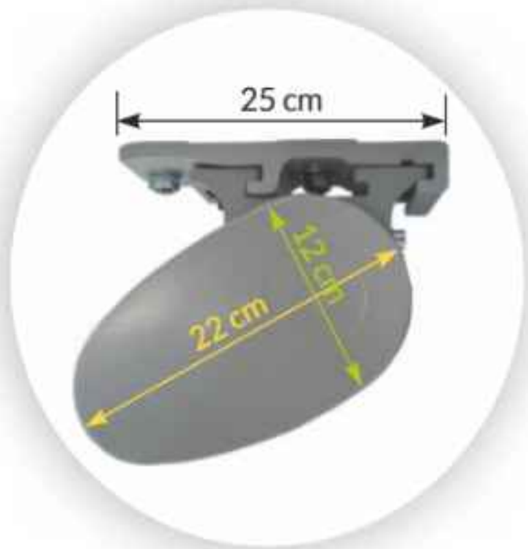
Deckenmontage
