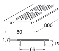
Ventilation grille
