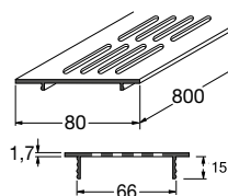
Ventilation grille
