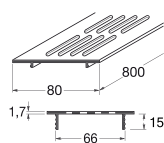
Ventilation grille
