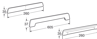
exclusiv end caps
