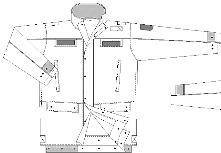
Abbildung 10 - technische Zeichnung Vorderteil
