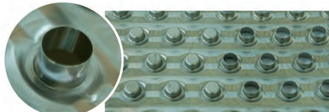
变薄拉伸结构 Drawless Type
