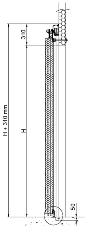
Threshold «SS»
