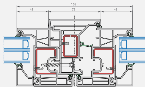
Horizontalschnitt
