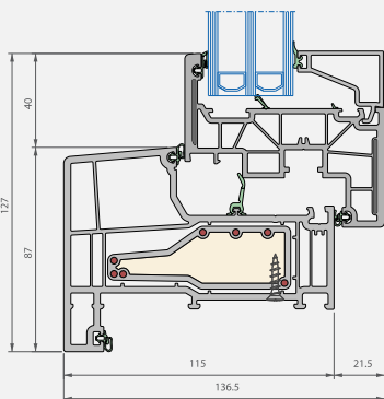
Vertikalschnitt
