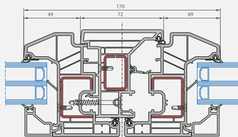
Horizontalschnitt
