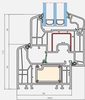
Vertikalschnitt
