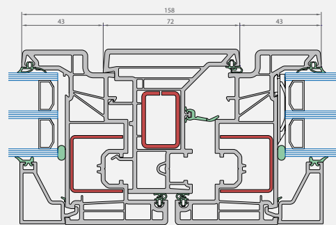
Horizontalschnitt
