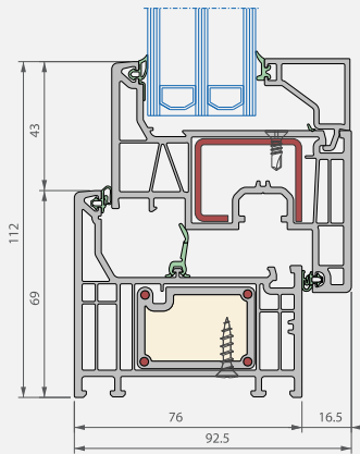
Vertikalschnitt
