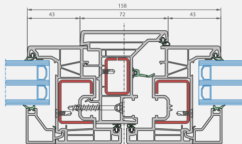
Horizontalschnitt
