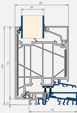
Vertikalschnitt
