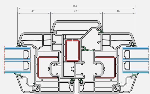
Horizontalschnitt
