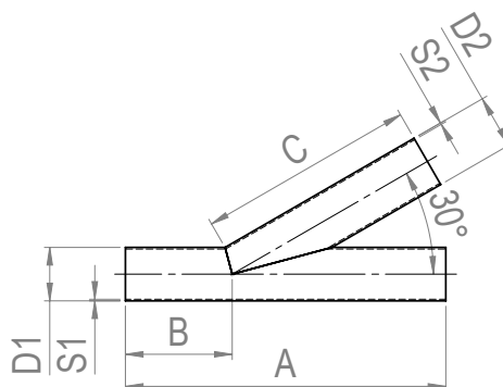
Edelstahl Abzweigstücke 30°
