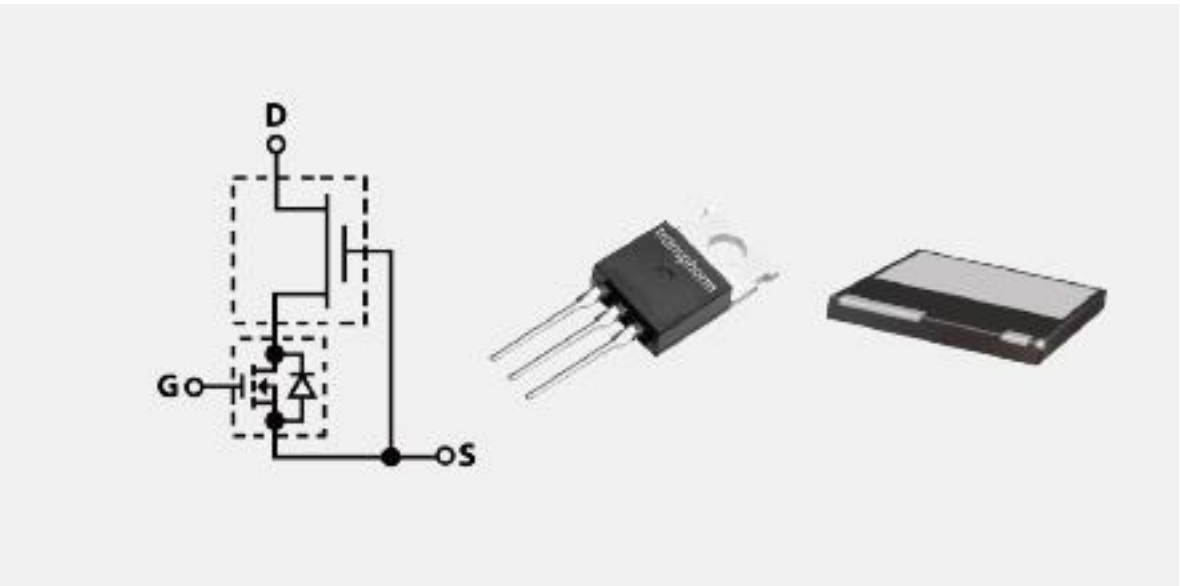
GaN HEMTs
