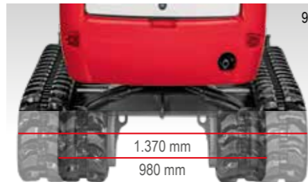
LAUFWERKSBEITRE
