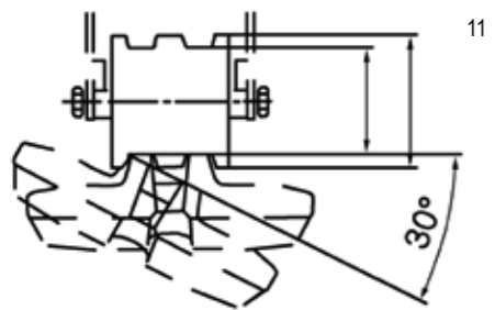
OPTIMALE KETTENFÜHRUNG
