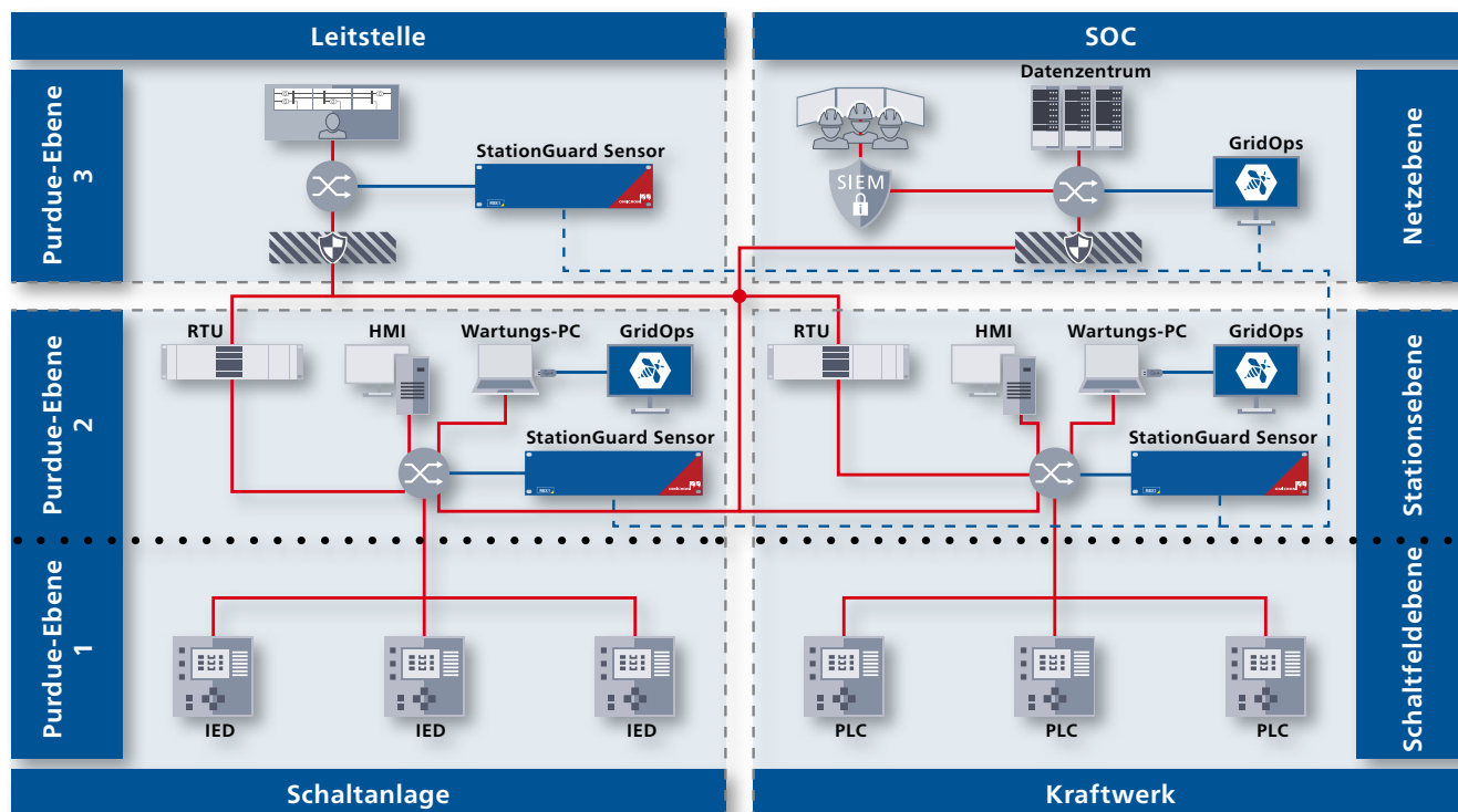
Integration von StationGuard in die Netzwerkinfrastruktur
