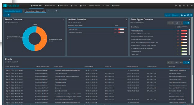
FortiSIEM-Integration
