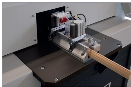
Pneumatische Werkstückklemmung
