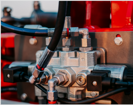
Elektrisches Umschaltventil
