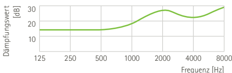
Dämpfungsverlauf
