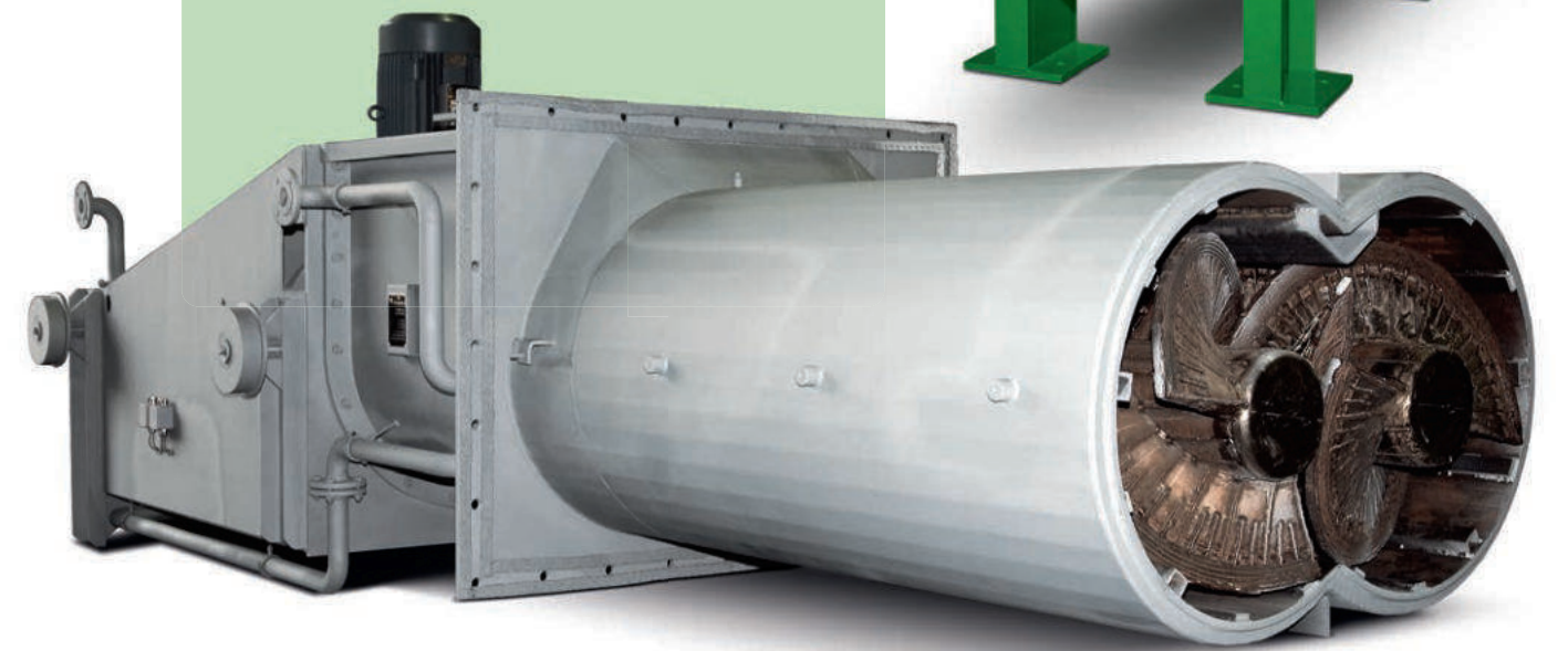
KÖLLEMAN Nickelierz-Hochtemperatur Eintragsschnecke
