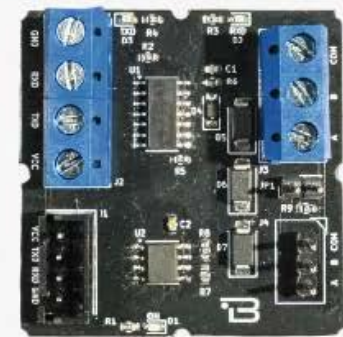
RS-485 Transceiver Module
