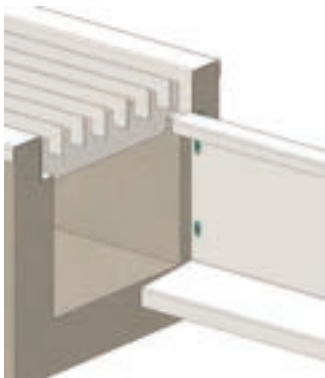
Anschluss Stopprinne
