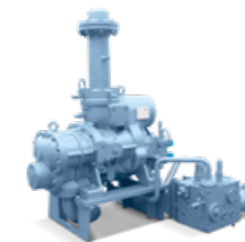
GEA Grasso Compressor Conversion Kit
