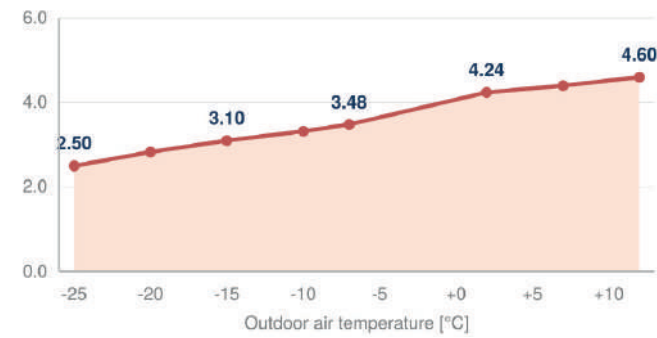
COP [-] — EN 14511-2
